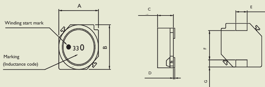
Dimensions : mm
